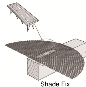
Shade Fix
