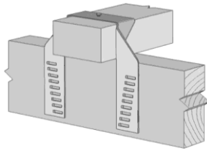
Batten Strap
